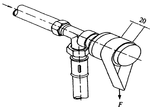
Рисунок 14. Испытание регулятора температуры на прочность при изгибе
