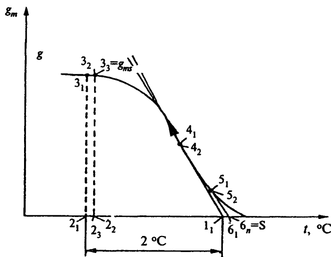
Рисунок 9. Расчет теоретической характеристики и точки S
