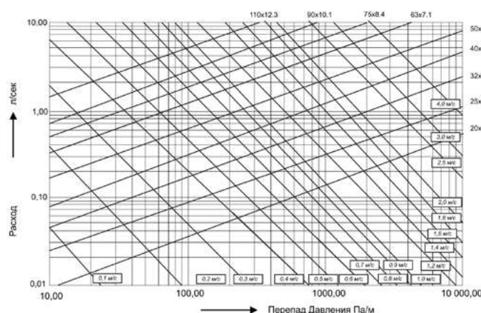
Номограмма потерь давления для труб РОСТерм FRP, армированных стекловолокном, SDR7,4/SDR9 при температуре 20 °C
