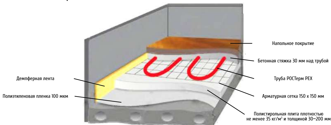
Разрез отопительной панели системы «Теплый пол» бетонного типа*
